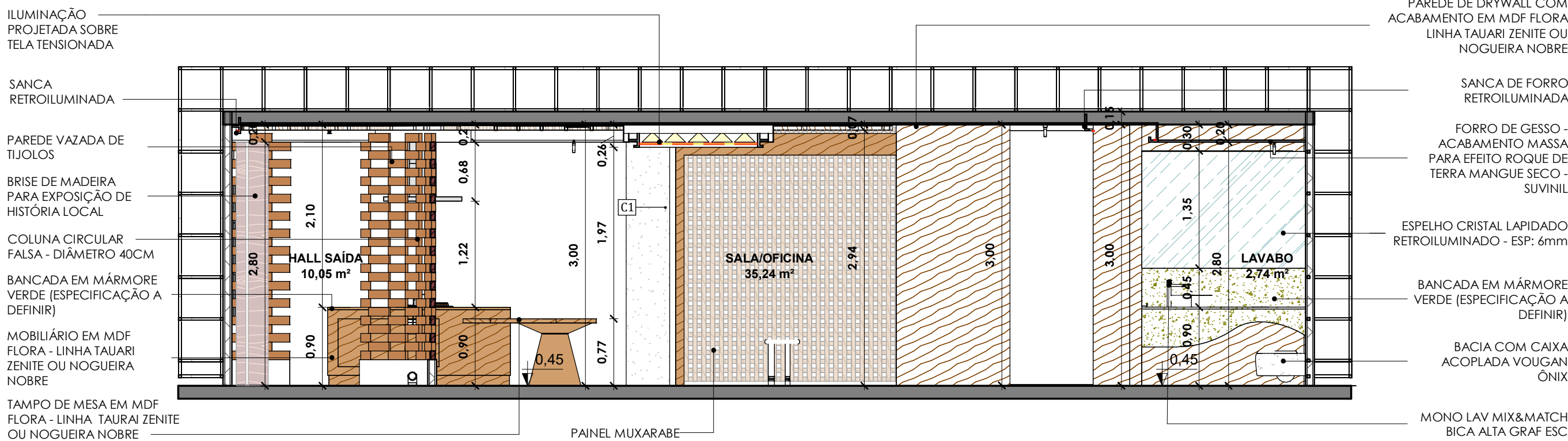
CORTE B 1 : 50
